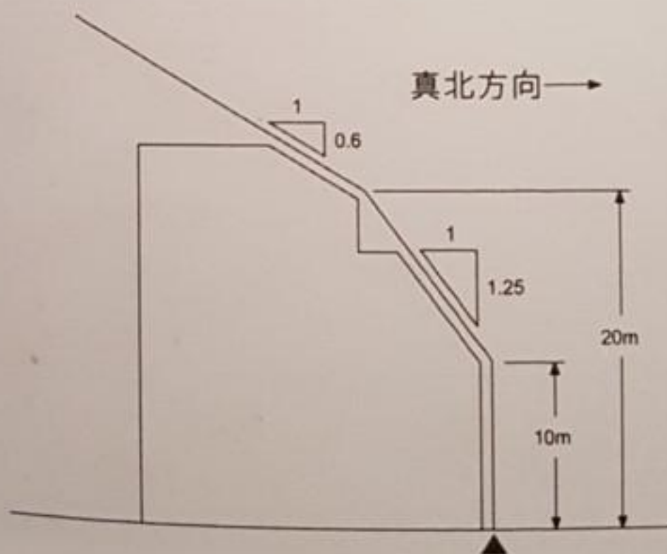
قانون مربوط به ارتفاع در ناحیه‌ی ۳ [توکیو]، شهرداری شیویا ۲
