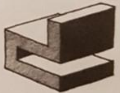
برش S نیمه half-S section
