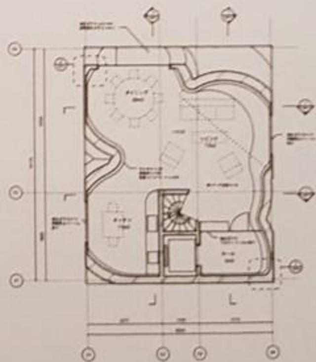
پلان طبقه‌ی چهارم
