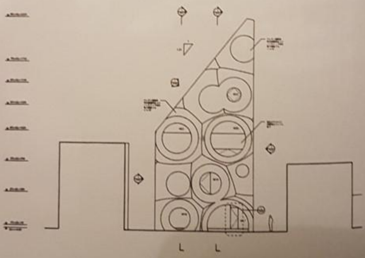
نمای غربی
